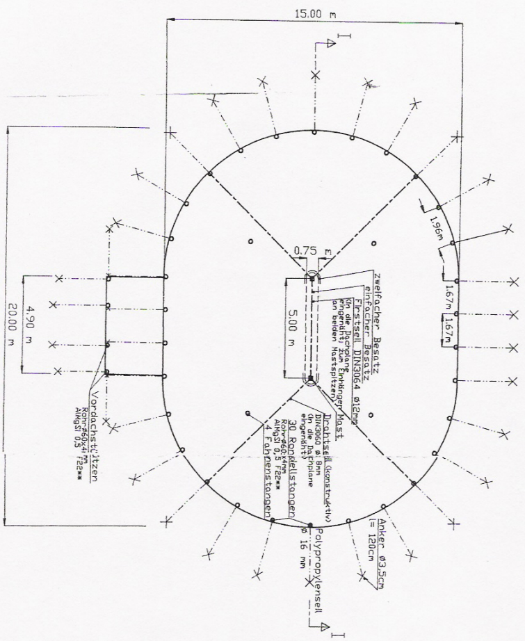
Anker und Planverstärkung nur im Grundriß dargestellt
